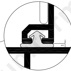
GUARNIZIONE DE04
