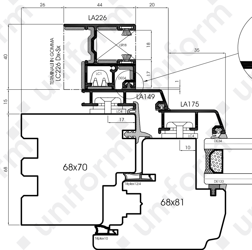
GUARNIZIONE DE04
